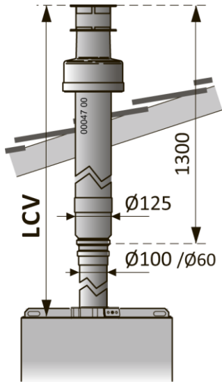
Приклад вертикальної системи (C 33 )
