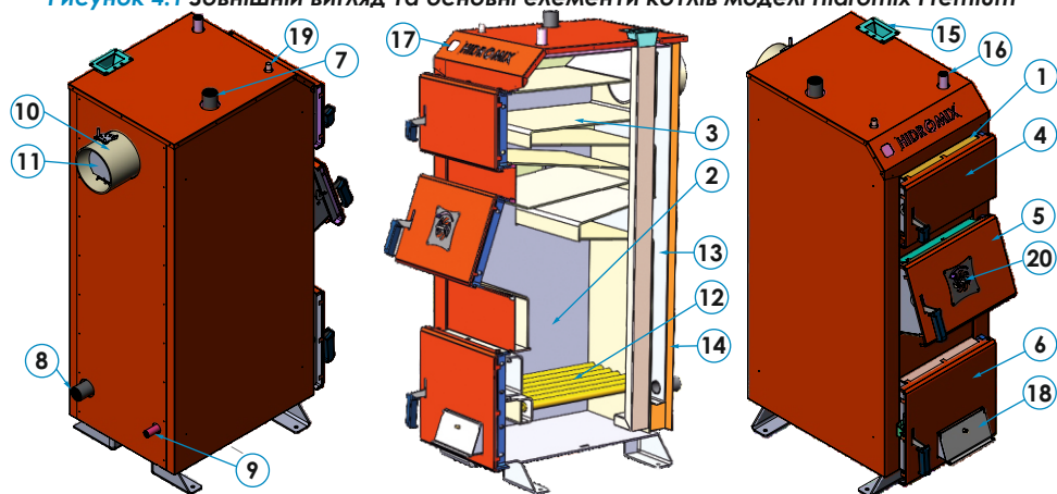
Рисунок 4.1 Зовнішній вигляд та основні елементи котлів моделі Hidromix Premium
