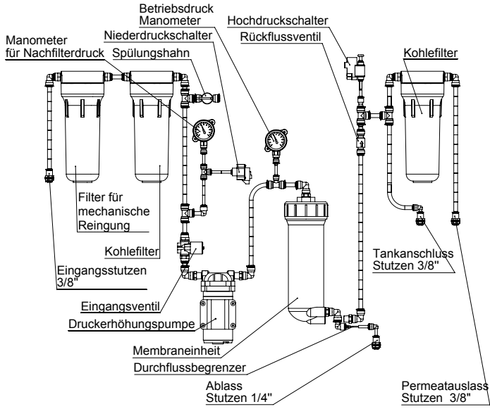
Abbildung 5. Schema des Systems RO ust 1500
