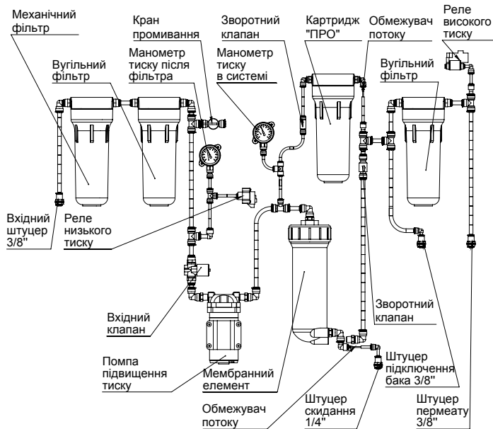
Рисунок 7. Схема системи Robust PRO (MO-1500)
