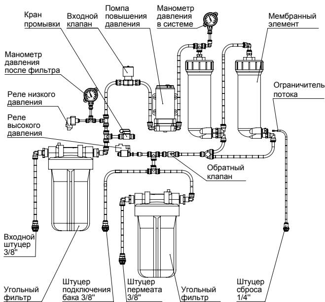
Рисунок 9. Схема системы ROBUST 3000
