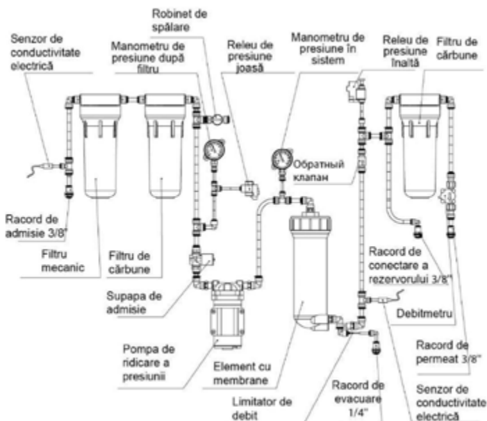
Figura 6. Schema sistemului ROust 1500 EC
