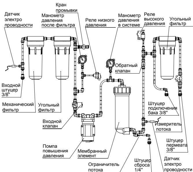
Рисунок 6. Схема системы ROBUST 1500 EC
