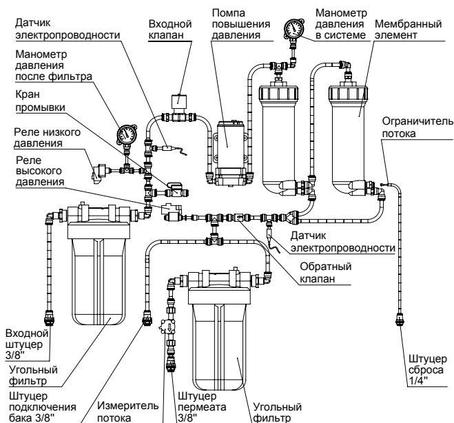
Рисунок 10. Схема системы ROBUST 3000 EC
