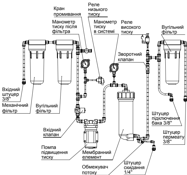
Рисунок 5. Схеми системи ROBUST 1500 (MO-1500)
