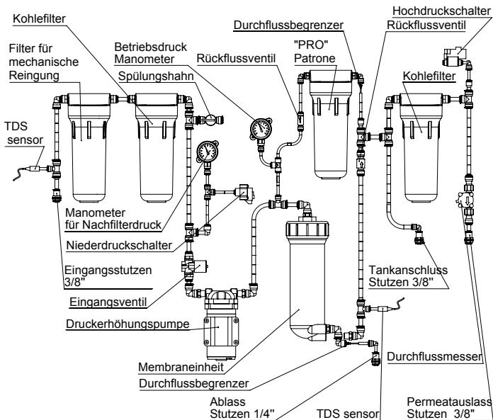
Abbildung 8. Schema des Systems Robust PRO EC
