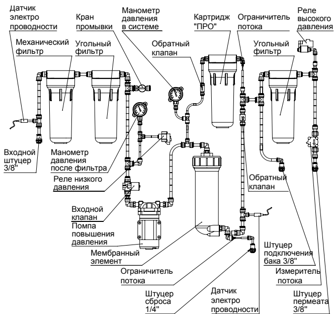
Рисунок 8. Схема системы ROBUST PRO EC
