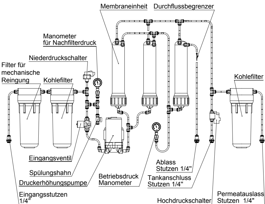
Abbildung 4. Schema des Systems Robust 1000
