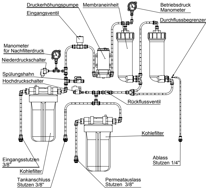
Abbildung 9. Schema des Systems ROBUST 3000
