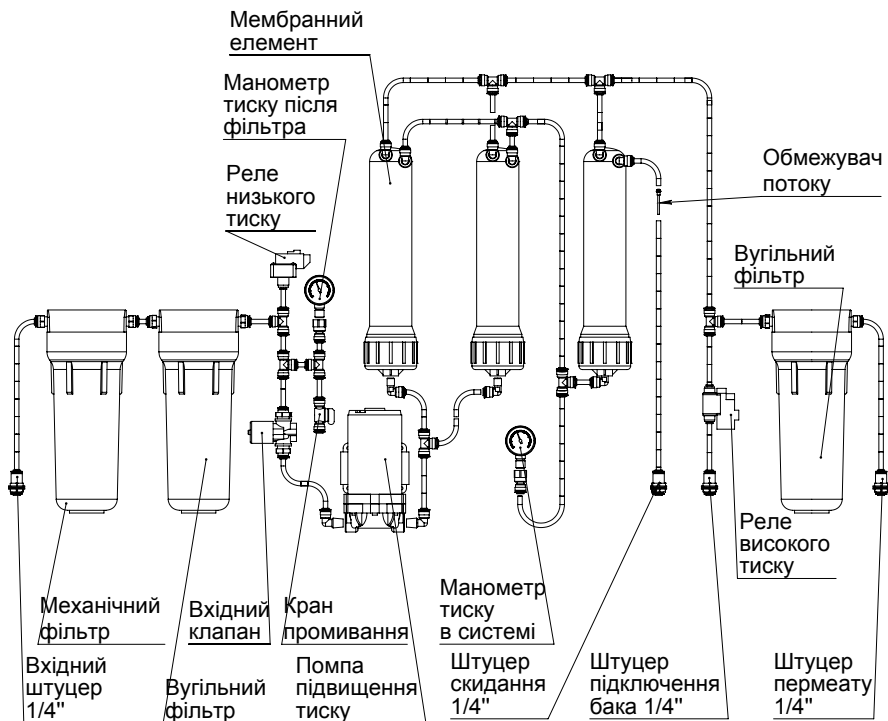
Рисунок 4. Схема системи ROBUST 1000 (MO-800)
