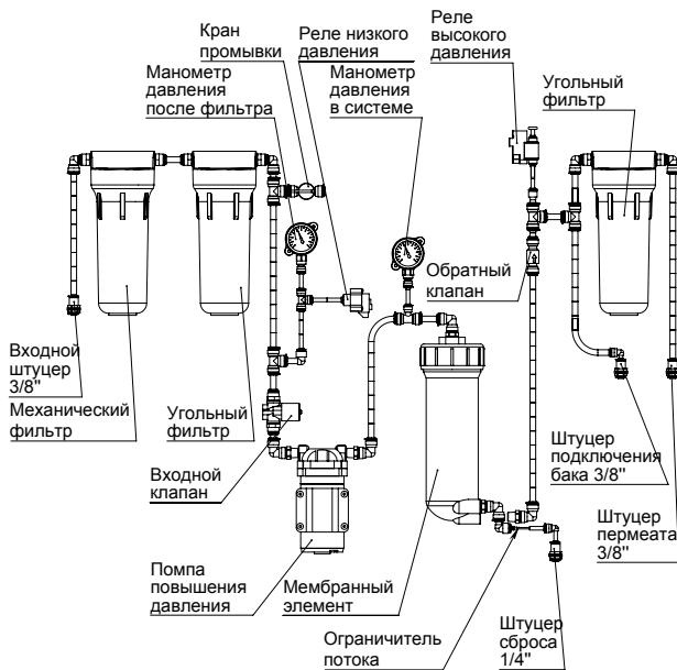
Рисунок 5. Схема системы ROBUST 1500
