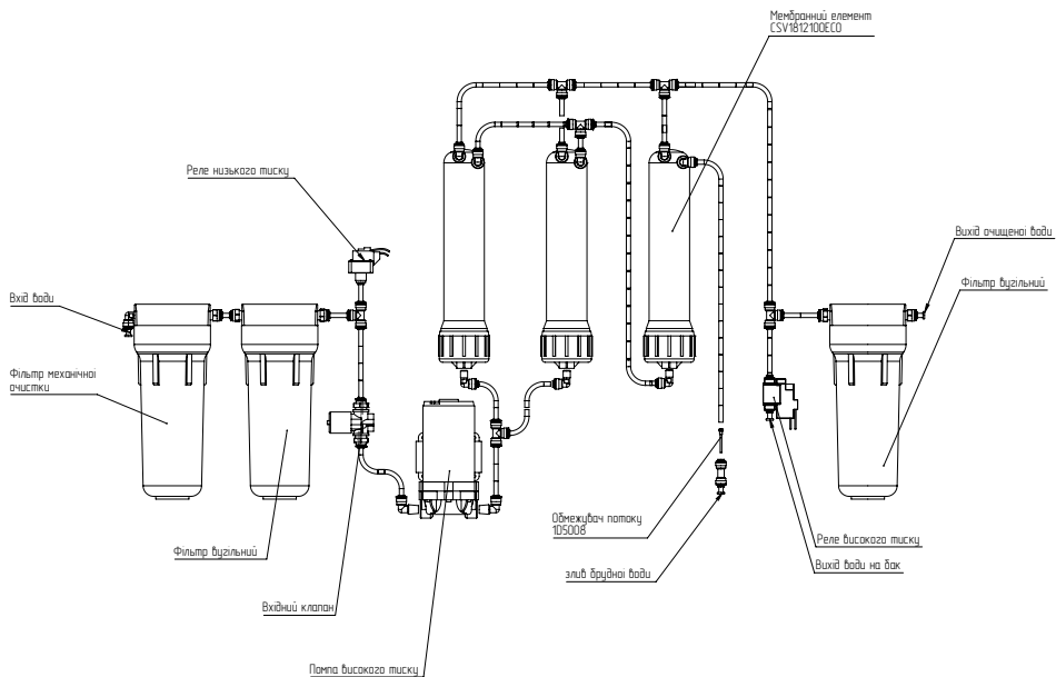
Figure 2. Robust Mini
