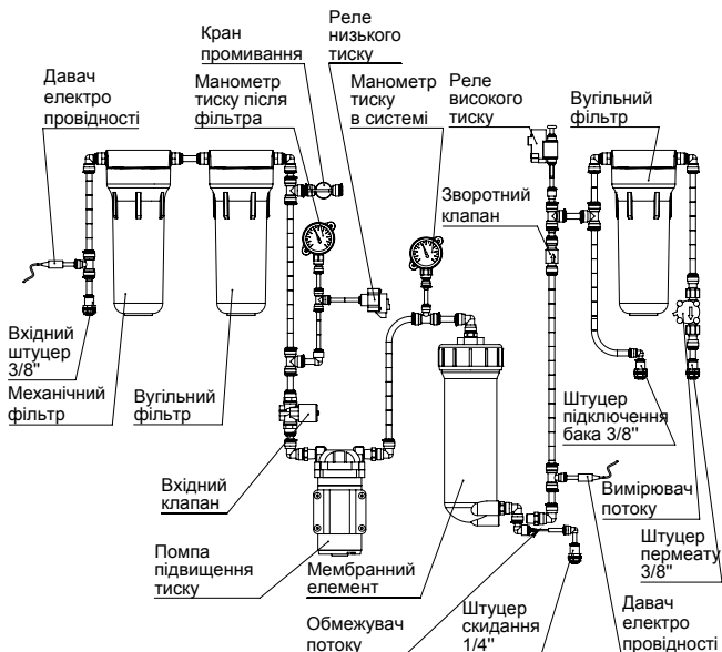
Рисунок 6. Схеми системи ROBUST 1500 EC (MO-1500)
