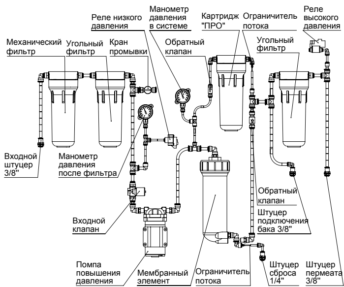
Рисунок 7. Схема системы ROBUST PRO
