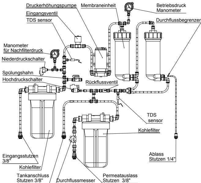
Abbildung 10. Schema des Systems ROBUST 3000 EC
