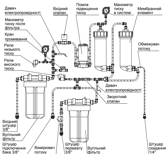
Рисунок 10. Схема системи ROBUST 3000 EC (MO-3000)
