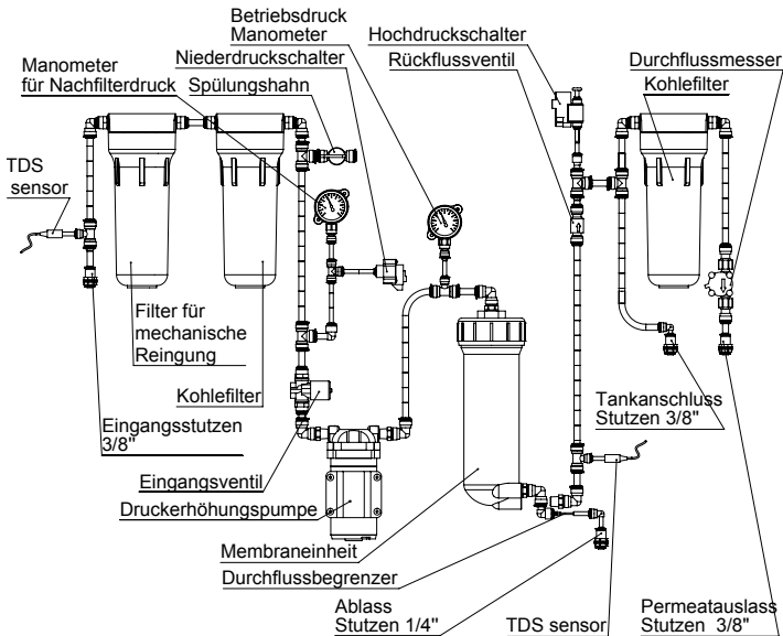
Abbildung 6. Schema des Systems RO ust 1500 EC
