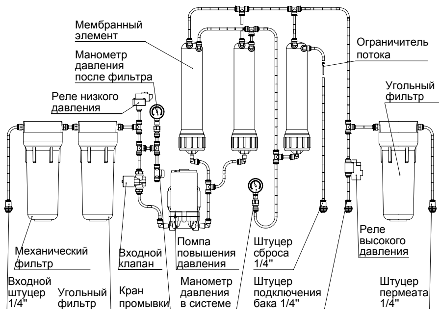
Рисунок 4. Схема системы ROust 1000
