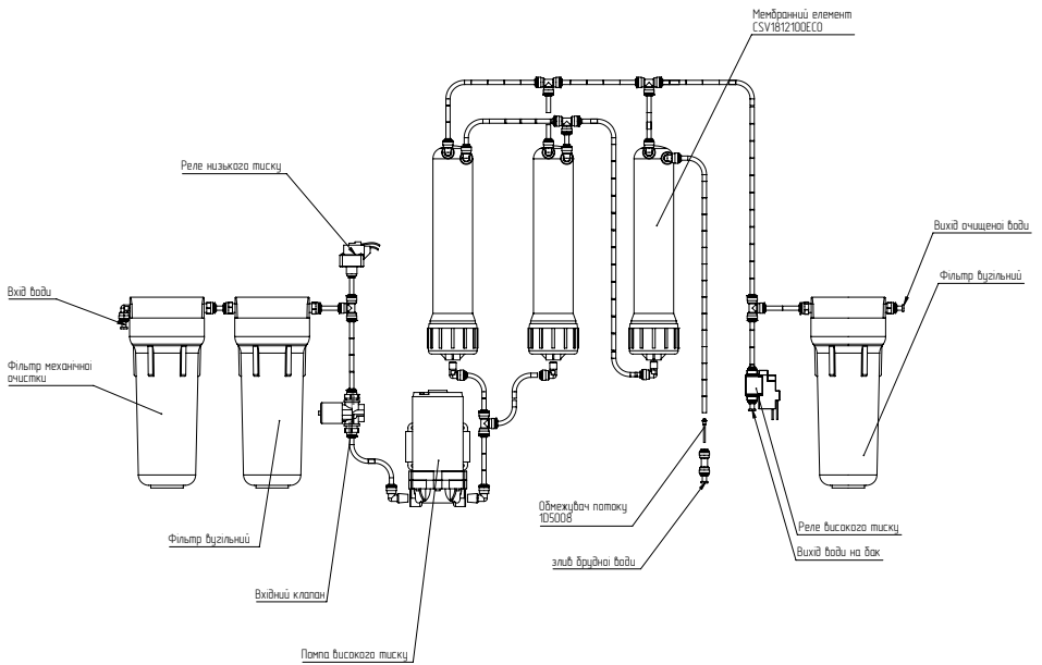
Figure 3. ROBust Mini
