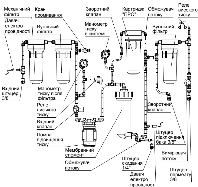
Рисунок 8. Схема системи Robust PRO EC (MO-1500)
