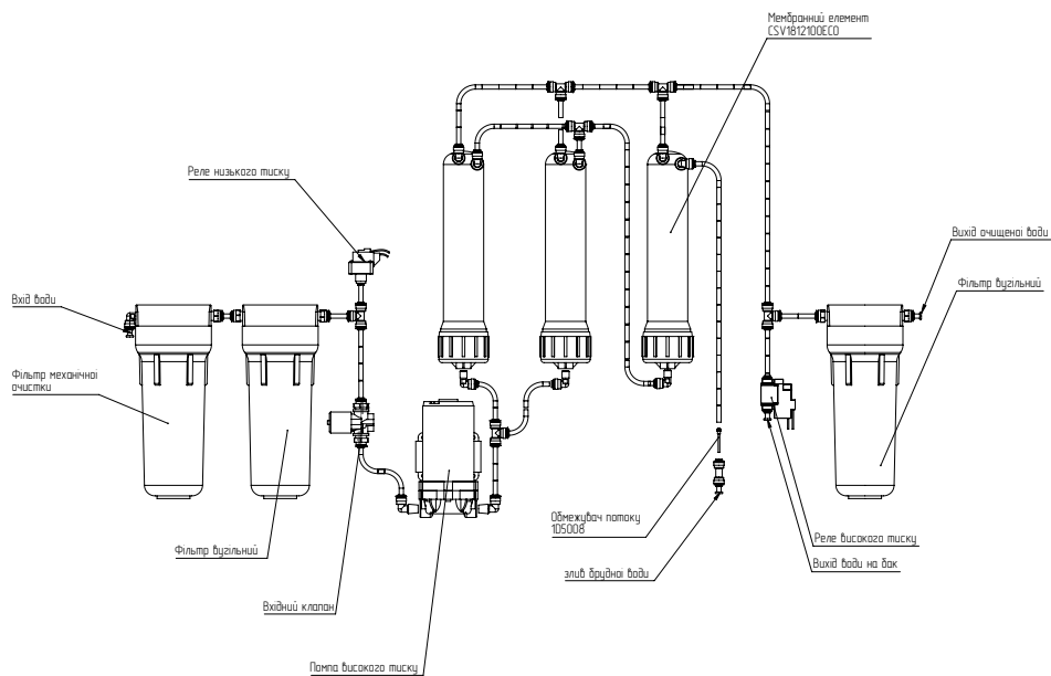
Figure 2. ROBUST Mini
