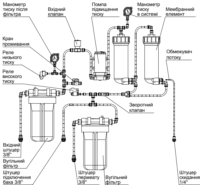
Рисунок 9. Схема системи ROBUST 3000 (MO-3000)
