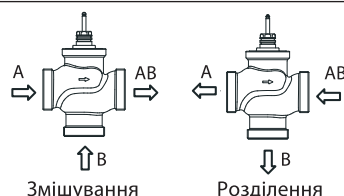
Мал.1. Підключення клапана VRB3 як змішувального, та як розділювального
