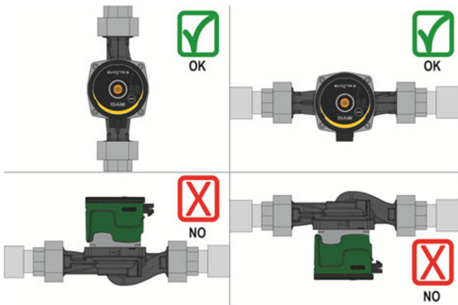
Εικόνα 3: Θέση συναρμολόγησης
